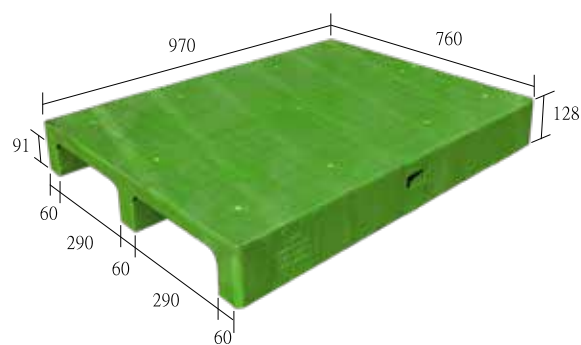
S2-9776-FG 一體成型
