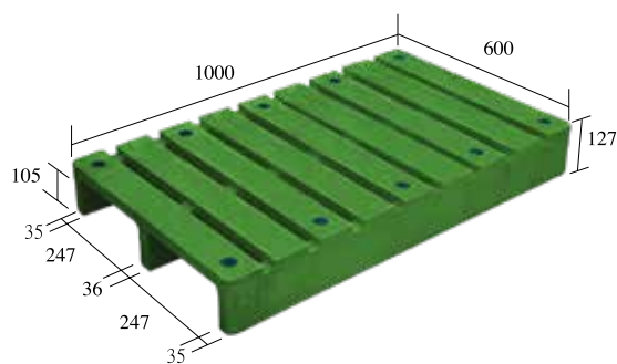
S2-1060-CG 一體成型
