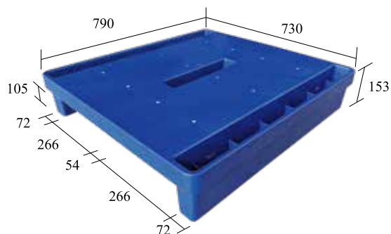
S2-7973-FG 一體成型
