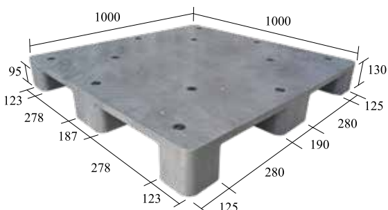
S4-1010-FG1 一體成型
