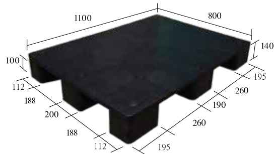
S4-1180-FG 一體成型
