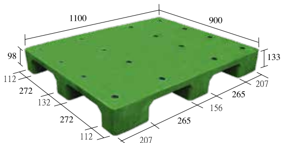
S4-1190-FG 一體成型
