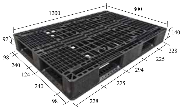
D4-1280-CG2 一體成型
