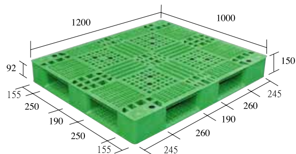
D4-1210-CG1 一體成型
