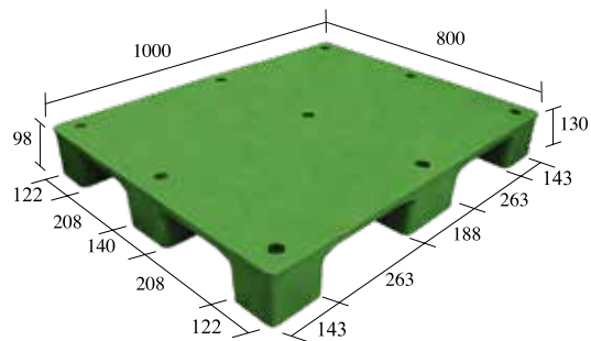
S4-1080-FG 一體成型
