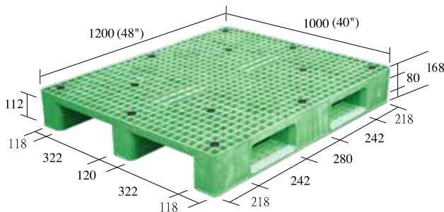
A4-1210-CX 一體成型
