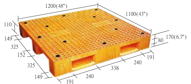
A4-1211-CX 一體成型
