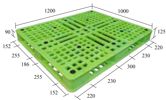
D4-1210-CG4 一體成型
