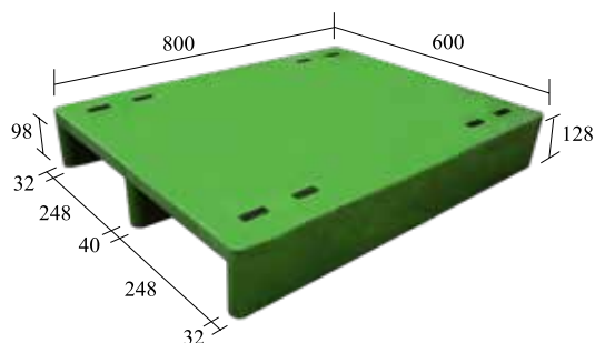
S2-8060-FG 一體成型
