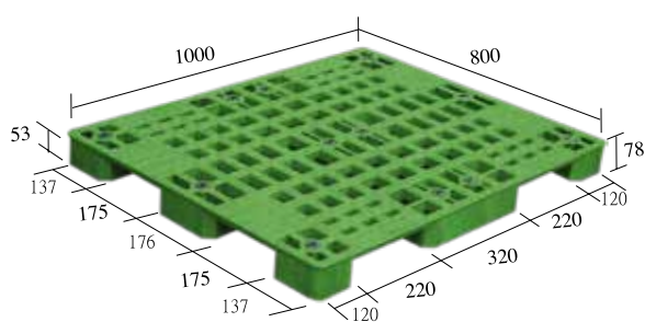
S4-1080-CG 一體成型
