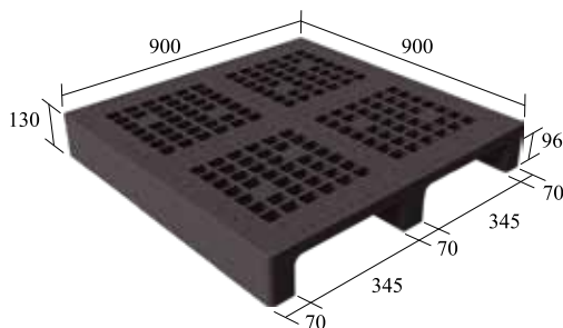
S2-9090-CG 一體成型
