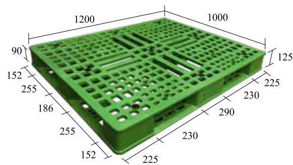
D4-1210-CG2 一體成型
