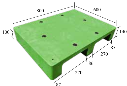
S2-8060-FG2 一體成型
