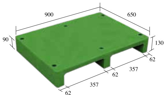
S2-9065-FG 一體成型
