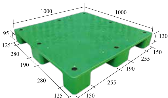
S4-1010-FG 一體成型
