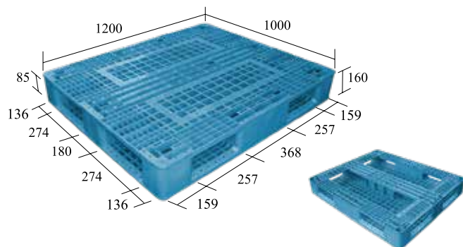
D4-1210-CG3 一體成型(日字型)
