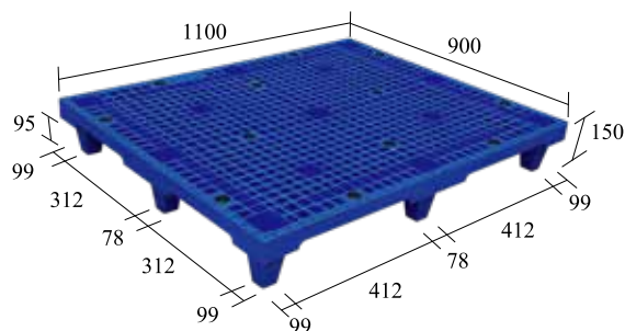
S4-1190-CE 一體成型
