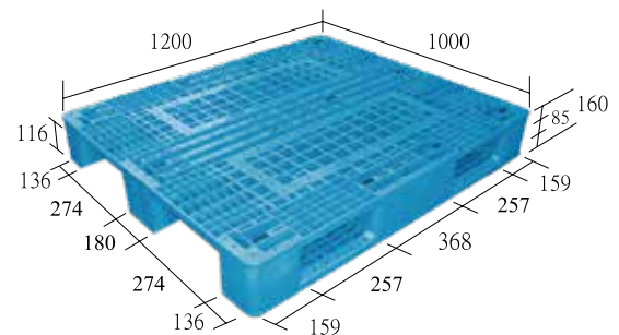
A4-1210-CG 一體成型
