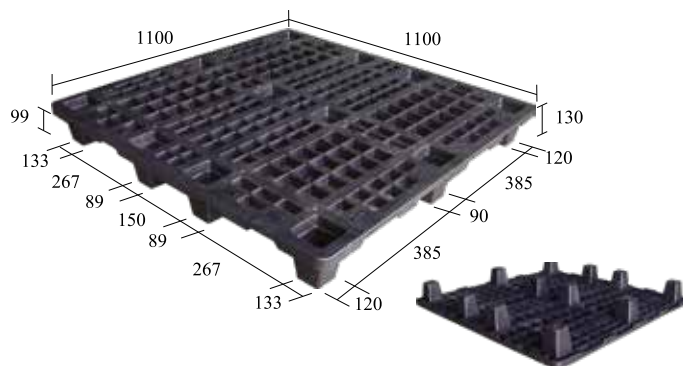
S4-1111-CE 一體成型 經濟型 NESTABLE
